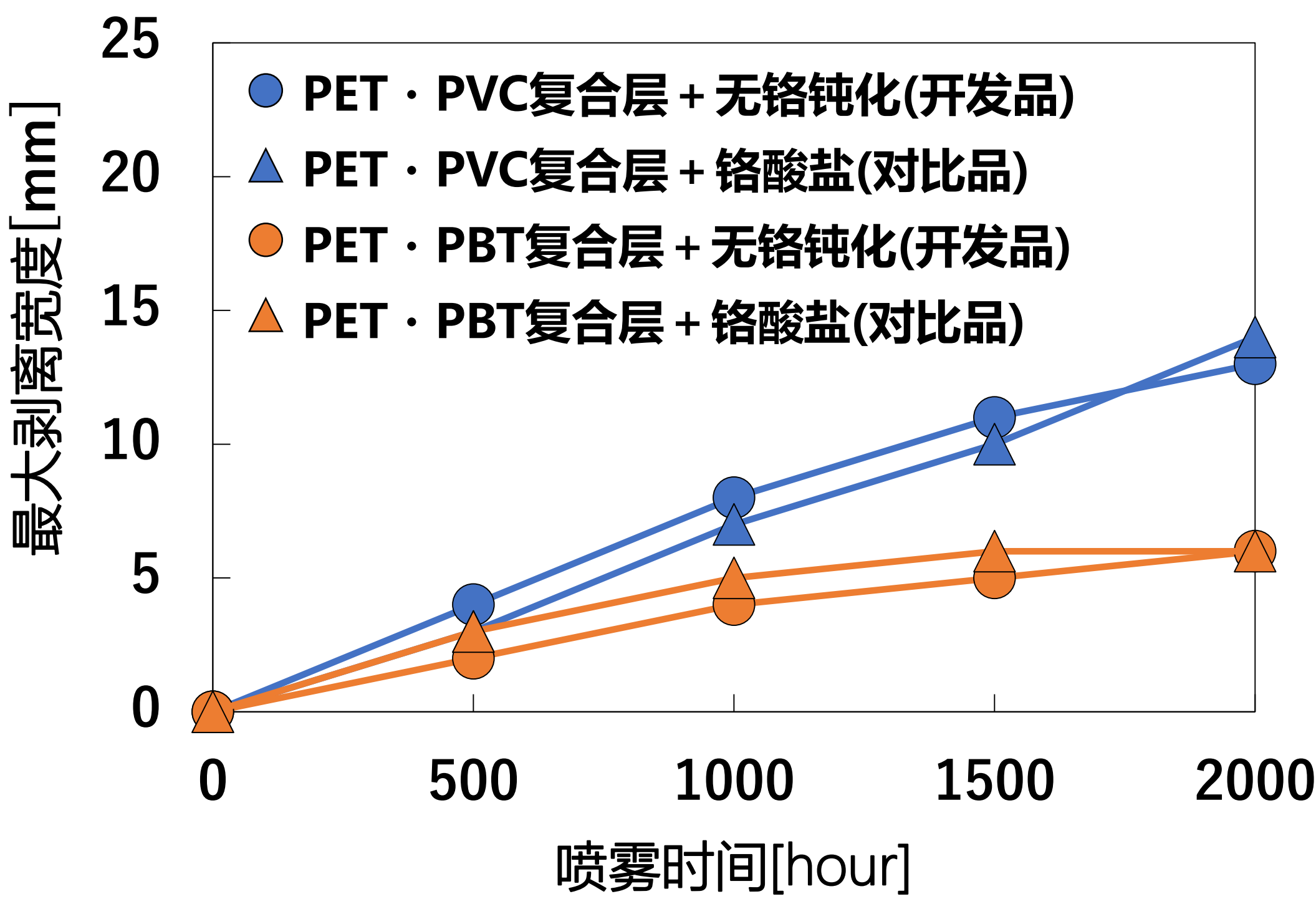
图2：耐食性试验结果※2
